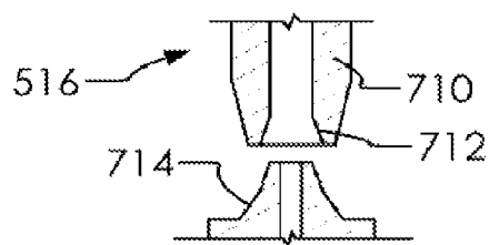
FIG. 7C
