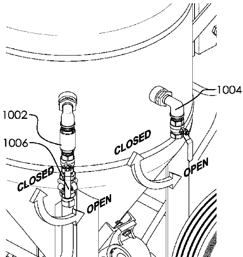
FIG. 10A
